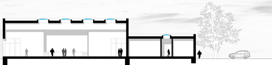
Schnitt D - D | m 1:400
